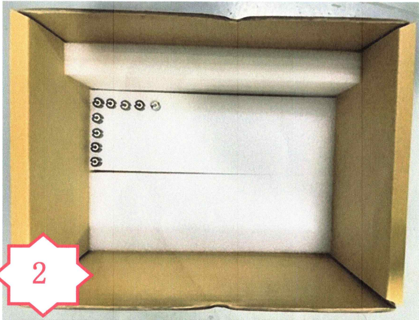
图二，将组件按图示装入箱内。一格 5 个，一层 20 格，放 4 层，一箱一共 400 个
